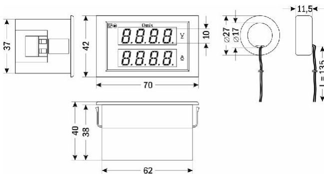
Рис. 2 – Размеры прибора
